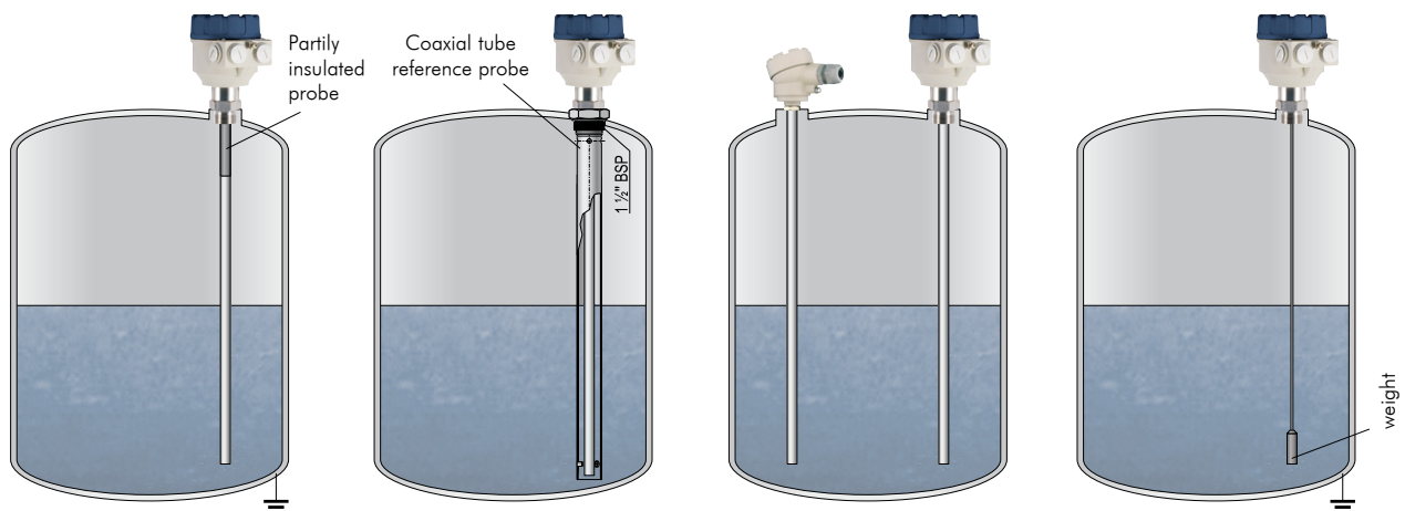
Rod probe
