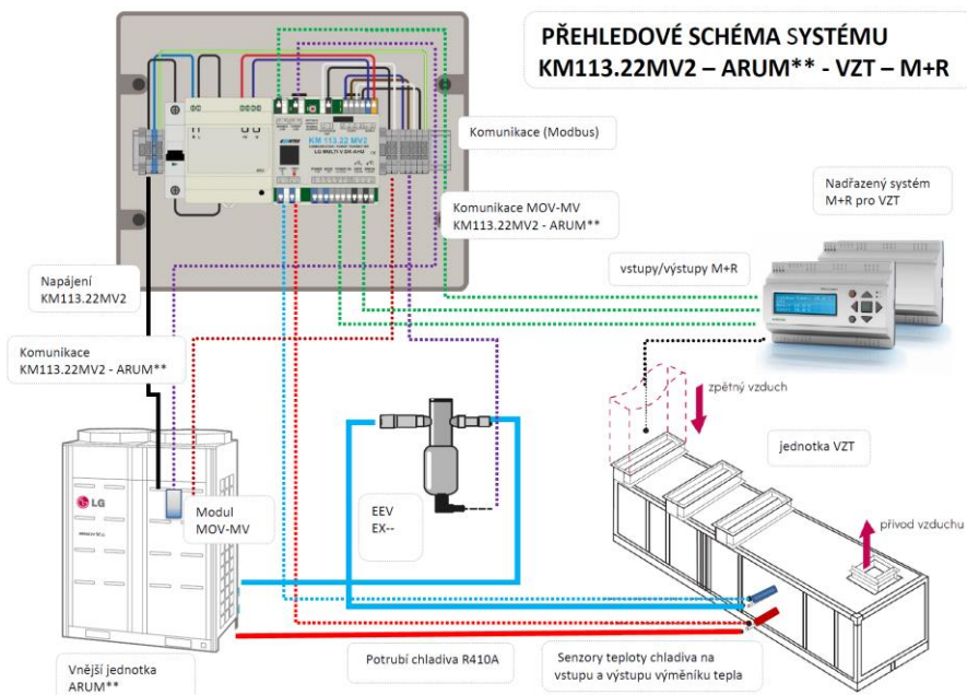
Obr. 1 PŘEHLEDOVÉ SCHÉMA APLIKACE
