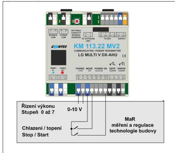
Obr.4 SCHÉMA OVLÁDÁNÍ VÝKONU ANALOGOVÝM SIGNÁLEM (PROVOZNÍ REŽIM OVLÁDÁNÍ LOGICKÝM VSTUPEM)
