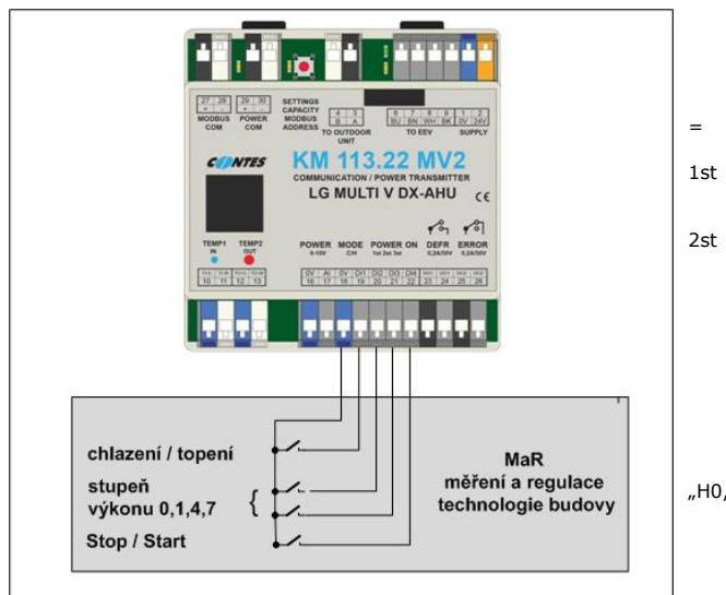
Obr.5 SCHEMA OVLÁDÁNÍ LOGICKÝMI SIGNÁLY - TYPU VOLNÝ KONTAKT
