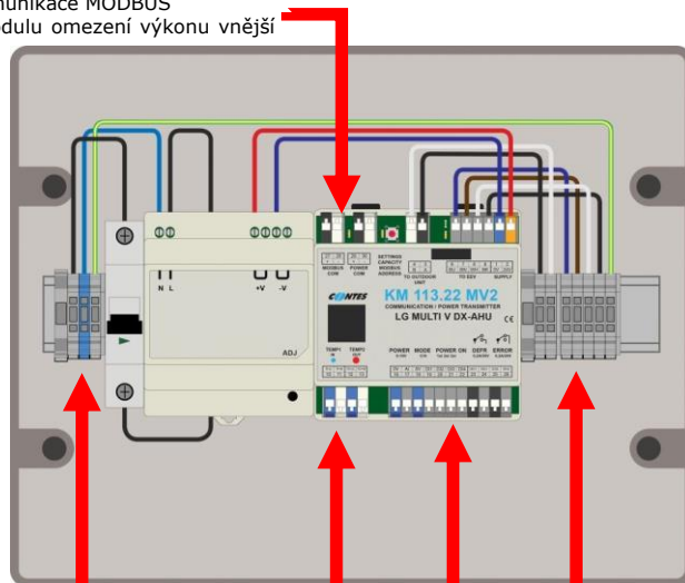
Obr. 3 ROZDĚLENÍ SVOREK MODULU KM113.22MV2
