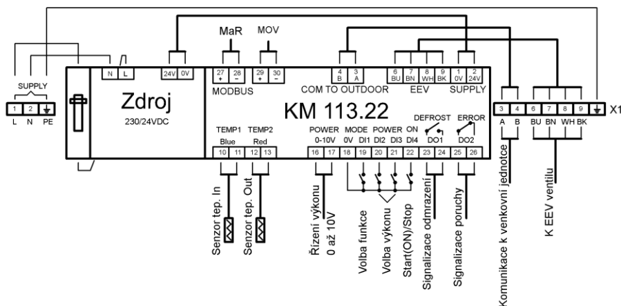
Obr. 2 CELKOVÉ SCHÉMA SVOREK
