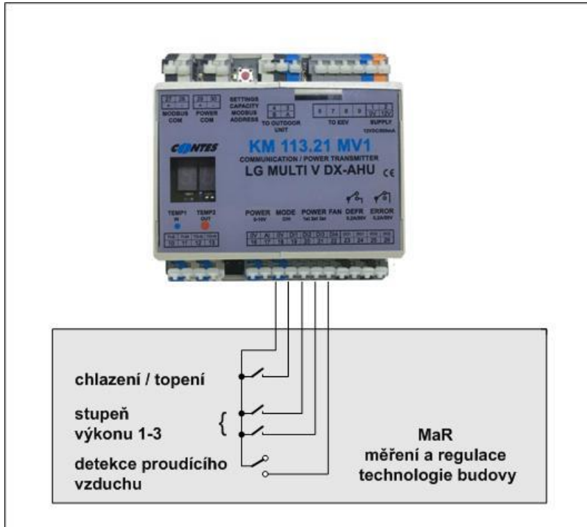
Obr.6 SCHEMA OVLÁDÁNÍ LOGICKÝMI SIGNÁLY - TYPU VOLNÝ KONTAKT
