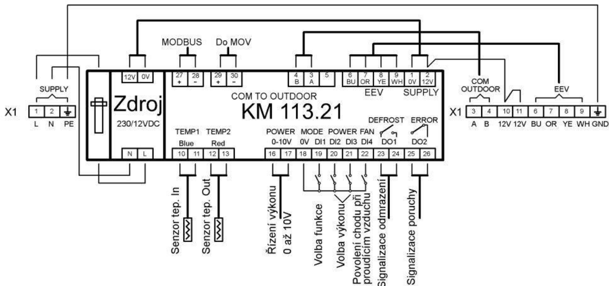
Obr. 3 CELKOVÉ SCHÉMA SVOREK
