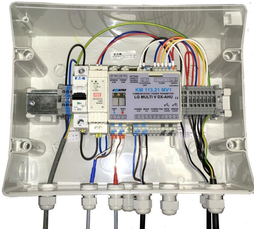
Obr. 4 PŘIPOJENÍ KABELŮ NAPÁJENÍ, SENZORŮ, VSTUPŮ A VÝSTUPŮ ZE SYSTÉMU M+R, KOMUNIKACE, A EEV
